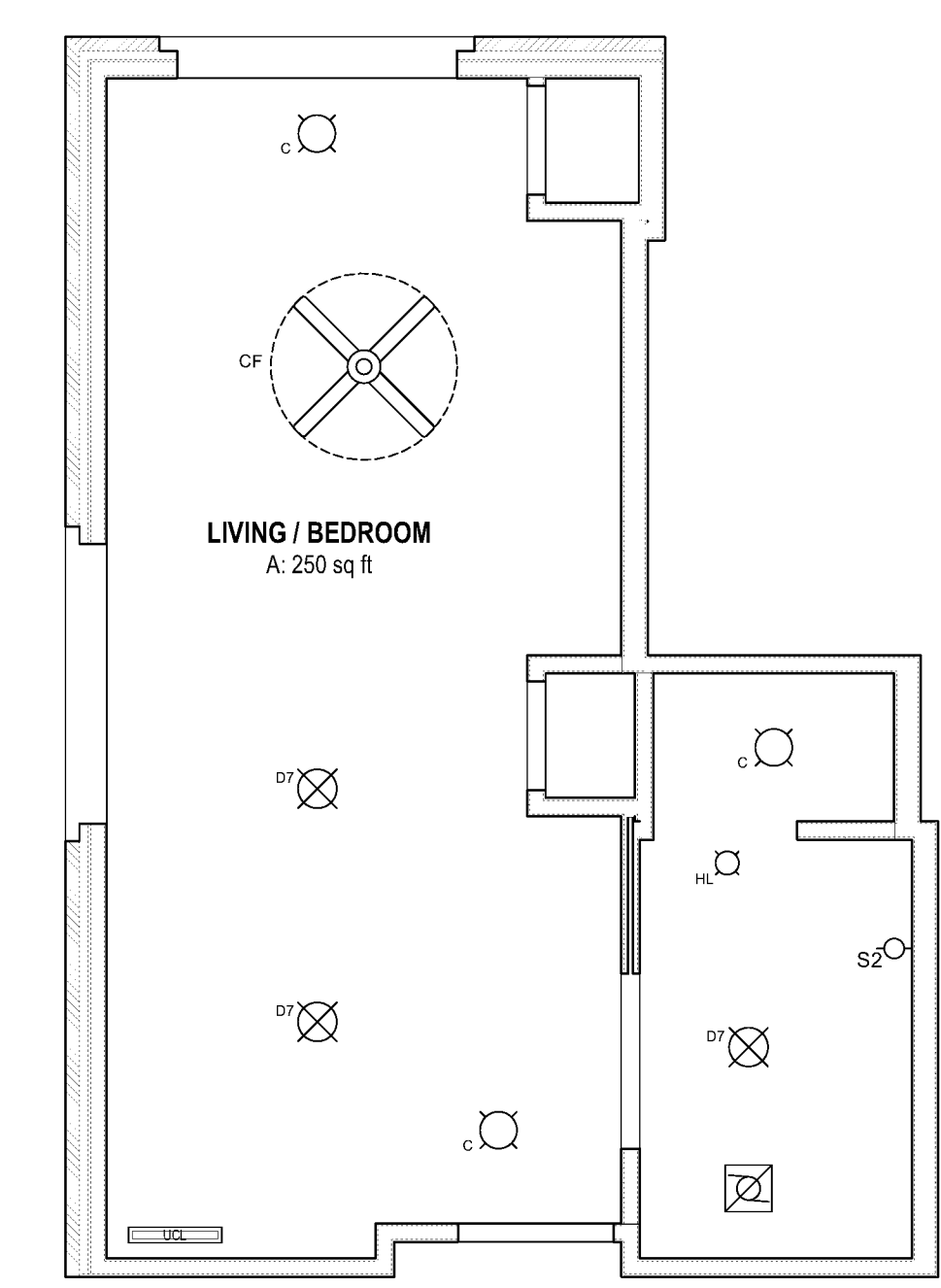
D5 UNIT RCP : MC-A4 STUDIO SCALE: 1/4" = 1'-0"
