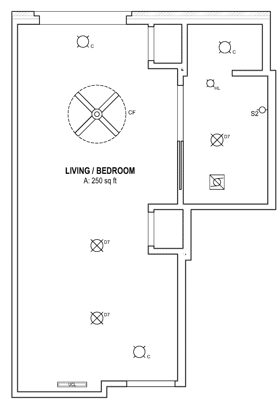
D2 UNIT RCP : MC-A2 STUDIO SCALE: 1/4" = 1'-0"
