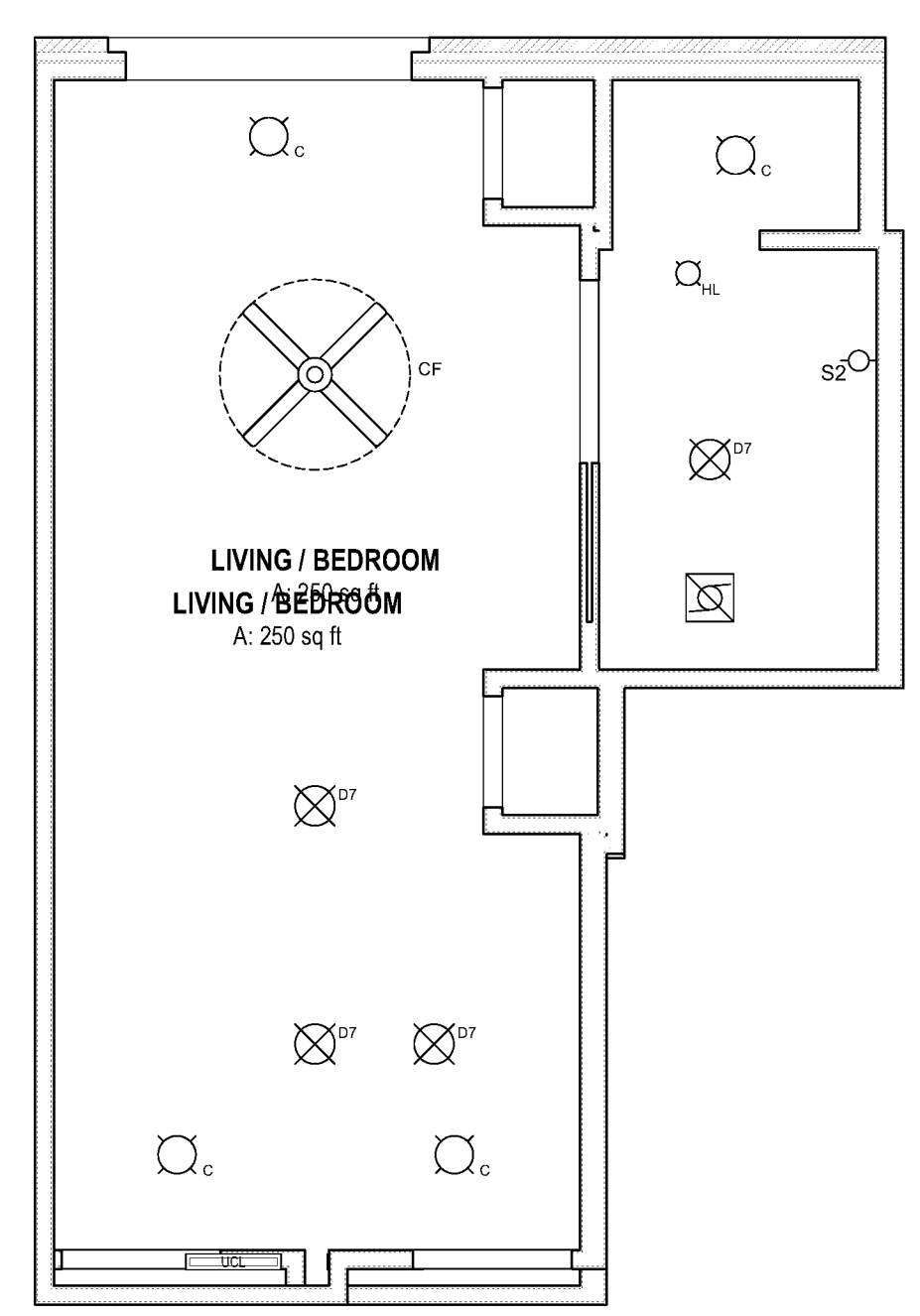
D1 UNIT RCP : MC-A2 STUDIO SCALE: 1/4" = 1'-0"
