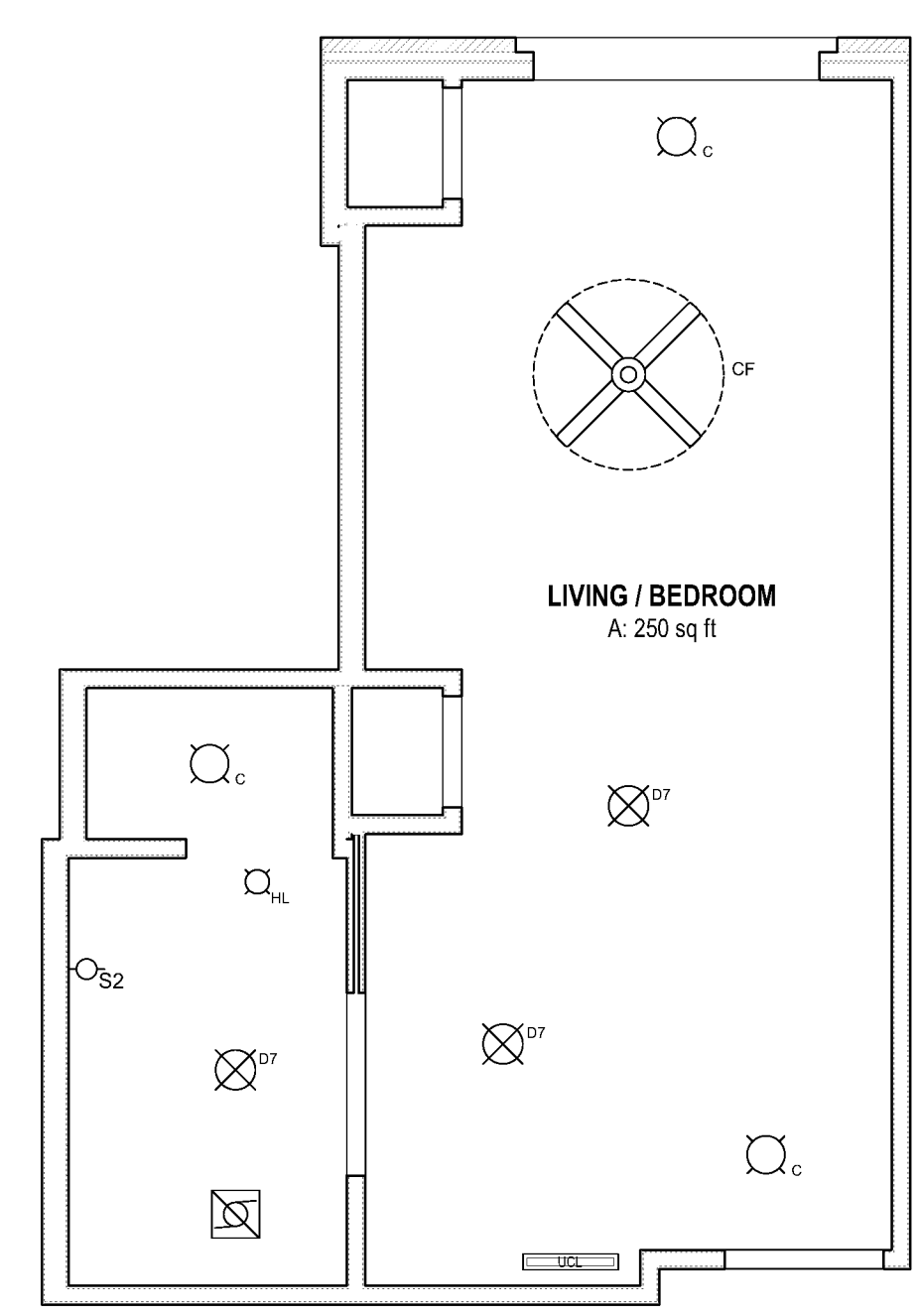
D3 UNIT RCP : MC-A3 STUDIO SCALE: 1/4" = 1'-0"
