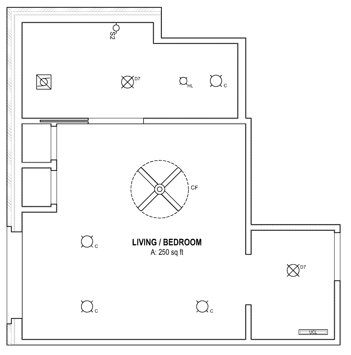
B1 UNIT RCP : MC-A4 STUDIO SCALE: 1/4" = 1'-0"
