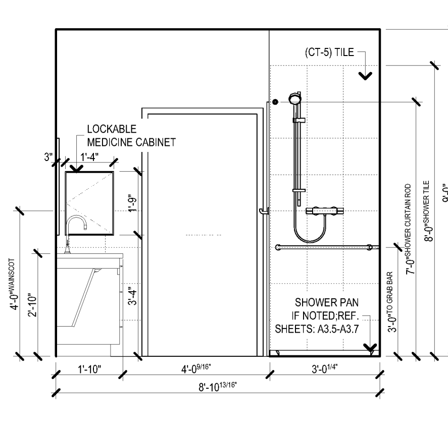
B3 AL TYPE 4 - BATHROOM SCALE: 3/8" = 1'-0"
