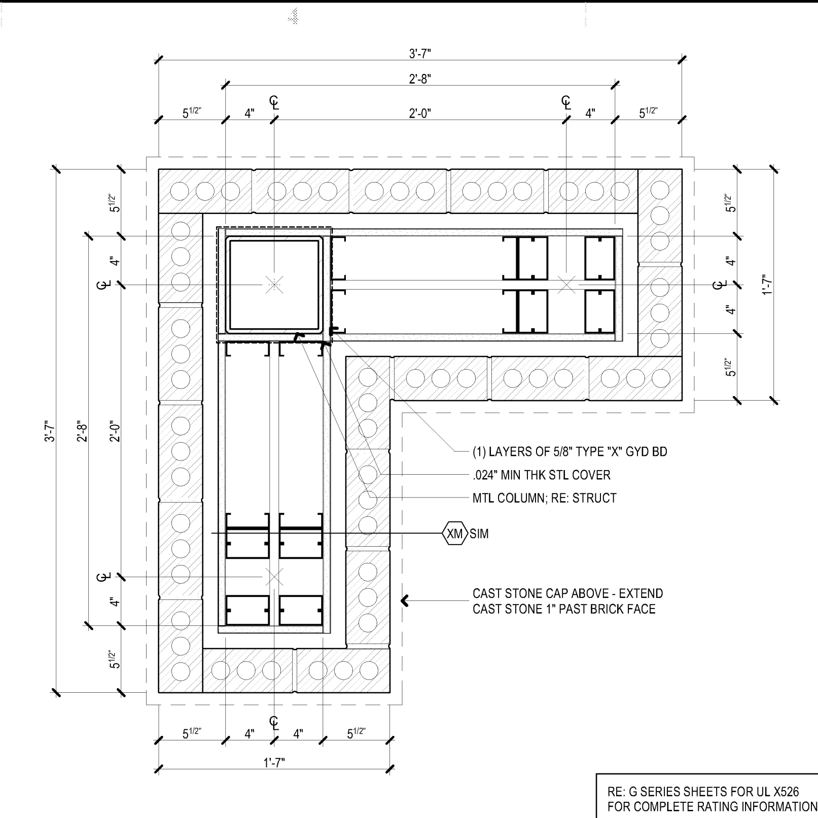
D4 PD PORTE COCHERE COLUMN DETAIL 01 SCALE: 1 1/2" = 1'-0"
