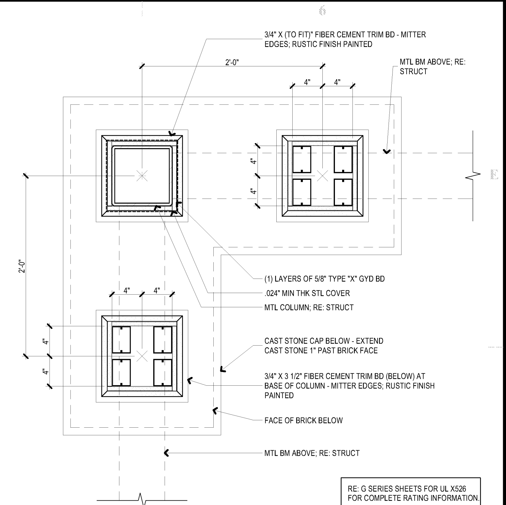
D5 PD PORTE COCHERE COLUMN DETAIL 02 SCALE: 1 1/2" = 1'-0"
