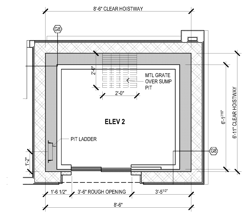
B5 ELEVATOR 2 - PIT PLAN SCALE: 3/8" = 1'-0"
