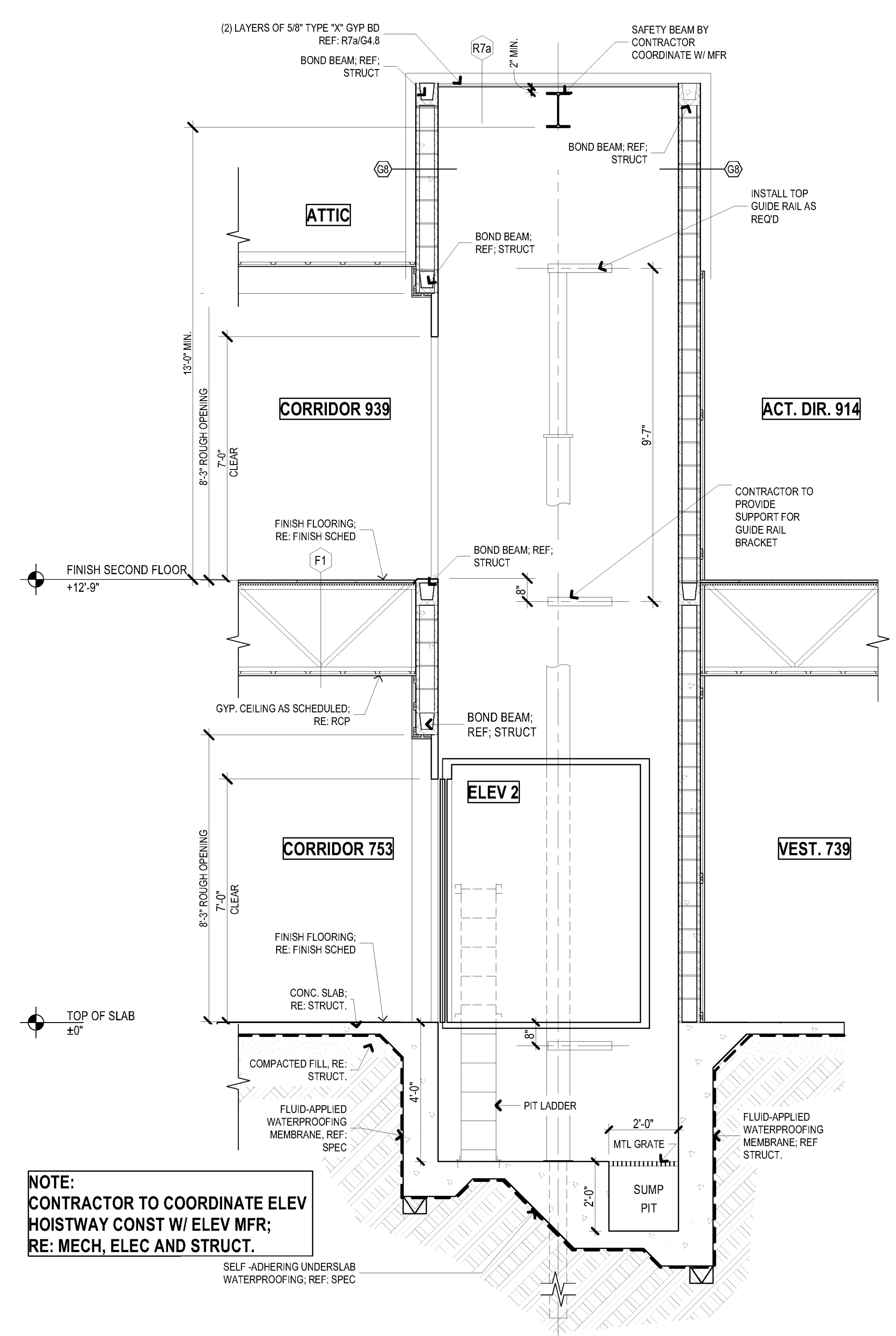
A3 SECTION - ELEVATOR 2 SCALE: 3/8" = 1'-0"
