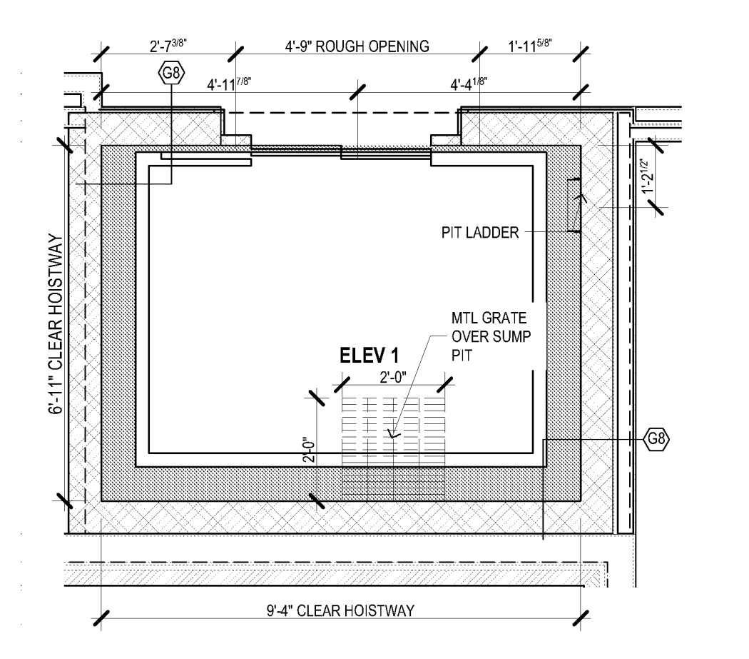
A5 ELEVATOR 1 - PIT PLAN SCALE: 3/8" = 1'-0"
