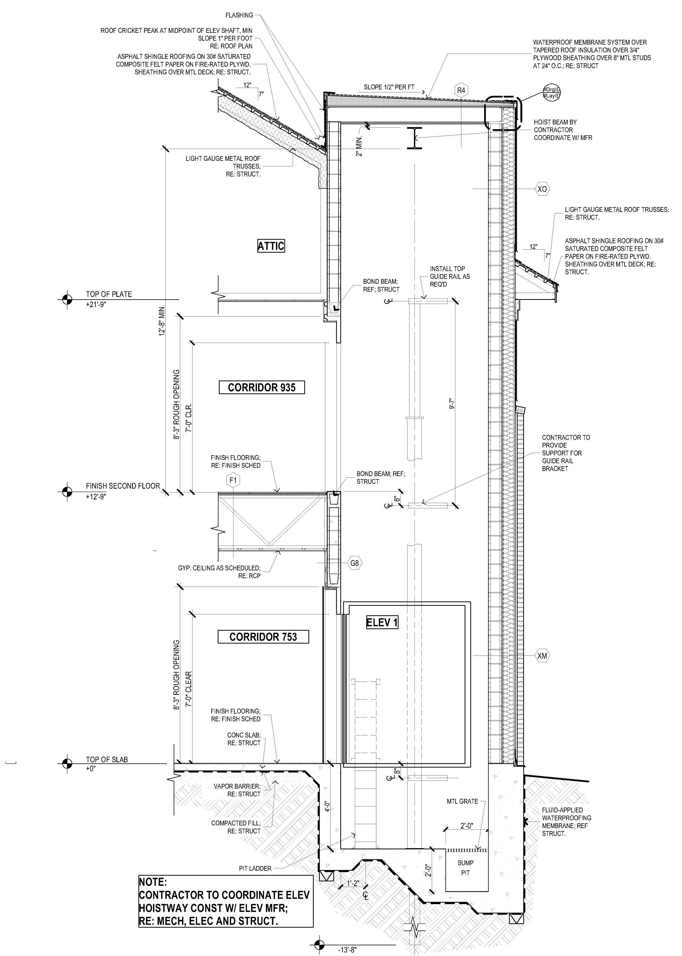
A1 SECTION - ELEVATOR 1 SCALE: 3/8" = 1'-0"
