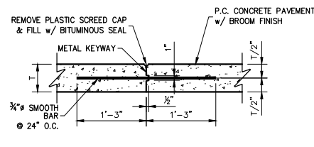
8 TYPICAL LONGITUDINAL JOINT "L" P.C. CONCRETE PAVEMENT SCALE: N.T.S.
