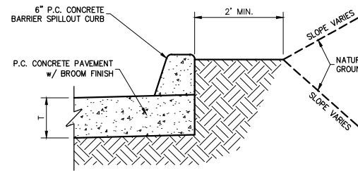
13 BACK OF CURB GRADING DETAIL SCALE: N.T.S.
