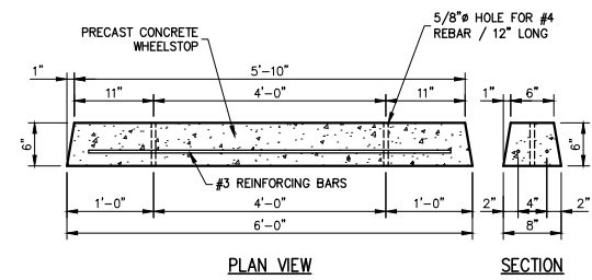
19 PRECAST CONCRETE WHEEL STOP SCALE: N.T.S.
